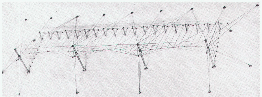
8 9 K. Melnikov, sowjetischer Pavillon auf der Internationalen Ausstellung in Paris, 1925. Perspektive und Grundrisse / Pavillon soviétique à l'exposition internationale de Paris. Perspective et plans / Soviet Pavilion at the International Exhibition in Paris, perspective view and plans
