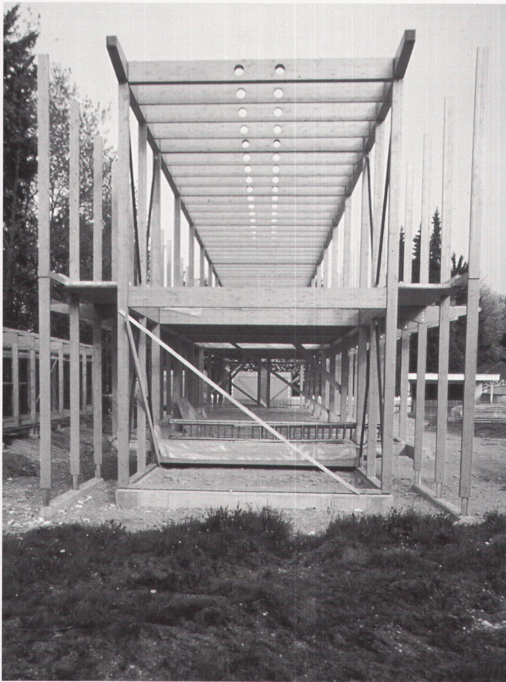
7 8 Montage der Holzkonstruktion
