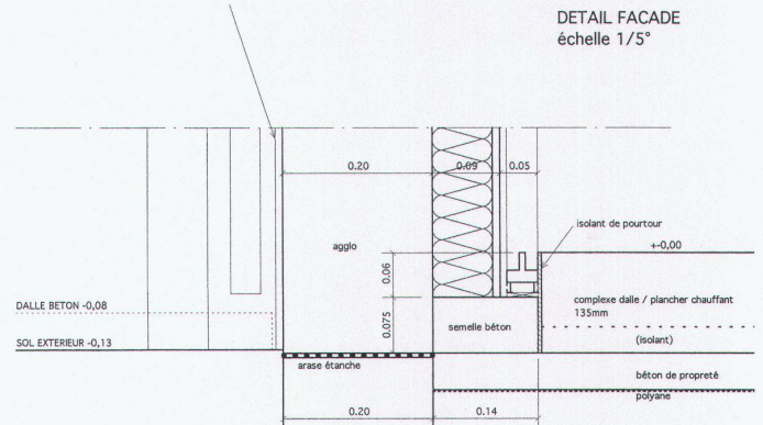
Detail geschlossene Wandpartie ▷ Détail de la partie pleine ▷ Detail of the closed wall section
