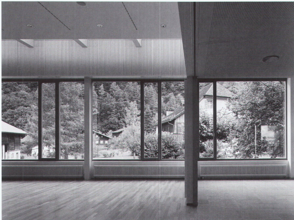
Foyer im Obergeschoss mit Verbindung zum Altbau
