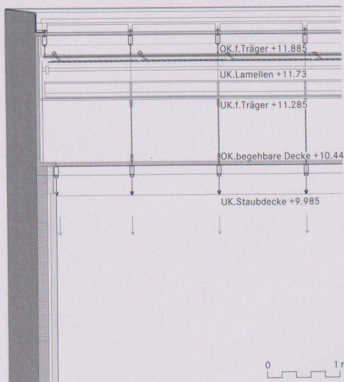
Detail Staubdecke
