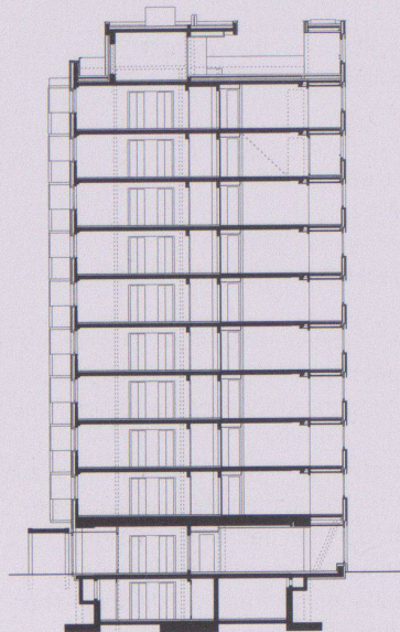
Schnitt
