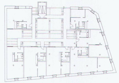
2. Obergeschoss
