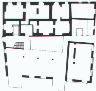
Erdgeschoss
