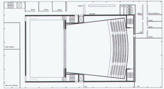
5. Obergeschoss
