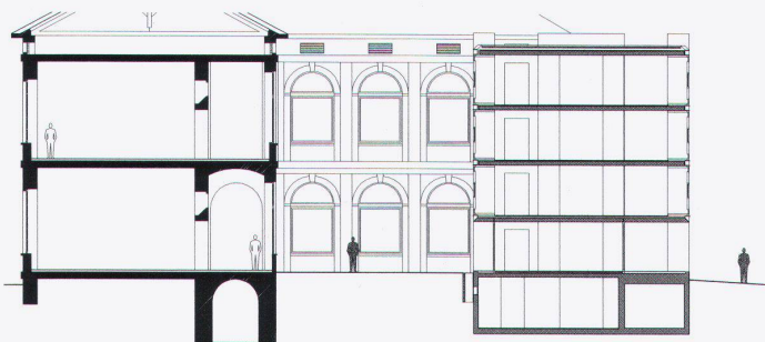
Bibliothek Schnitt
