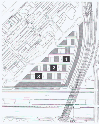
3, 4, 5 | NL-Architects: Het Funen, Reihenhauskomplex: Grundriss EG und Modelle
