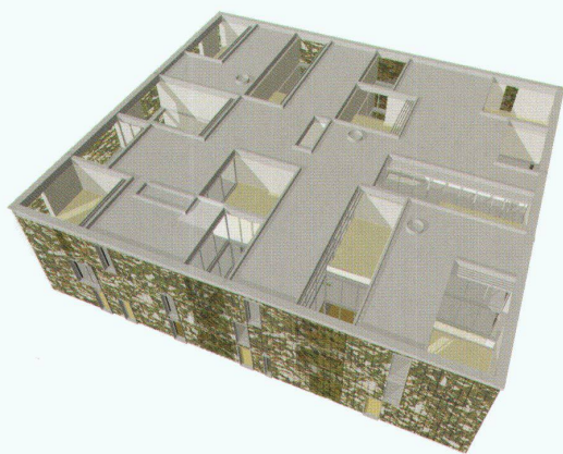
Geurst &amp; Schulze: Het Funen, Patiohäuser: Modell
