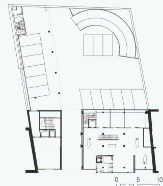
Erdgeschoss
