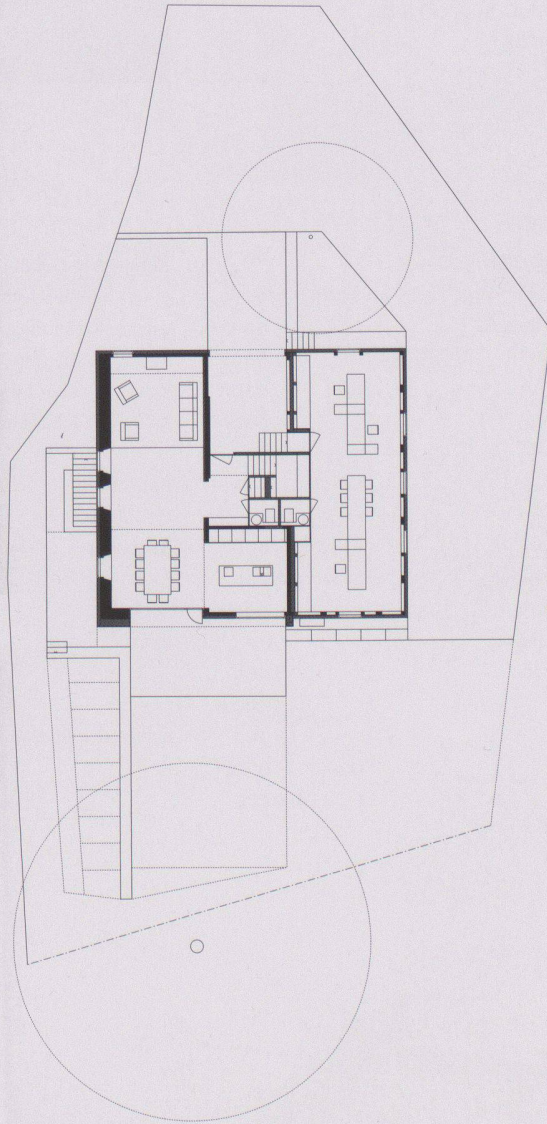
Grundriss 1.OG
