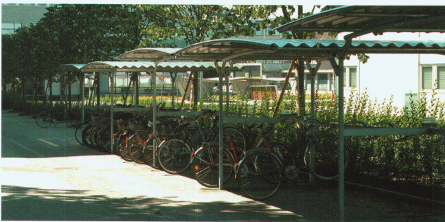
Möglichkeit von Dachversätzen bei Geländegefälle. Überdachung einseitig, offen.
