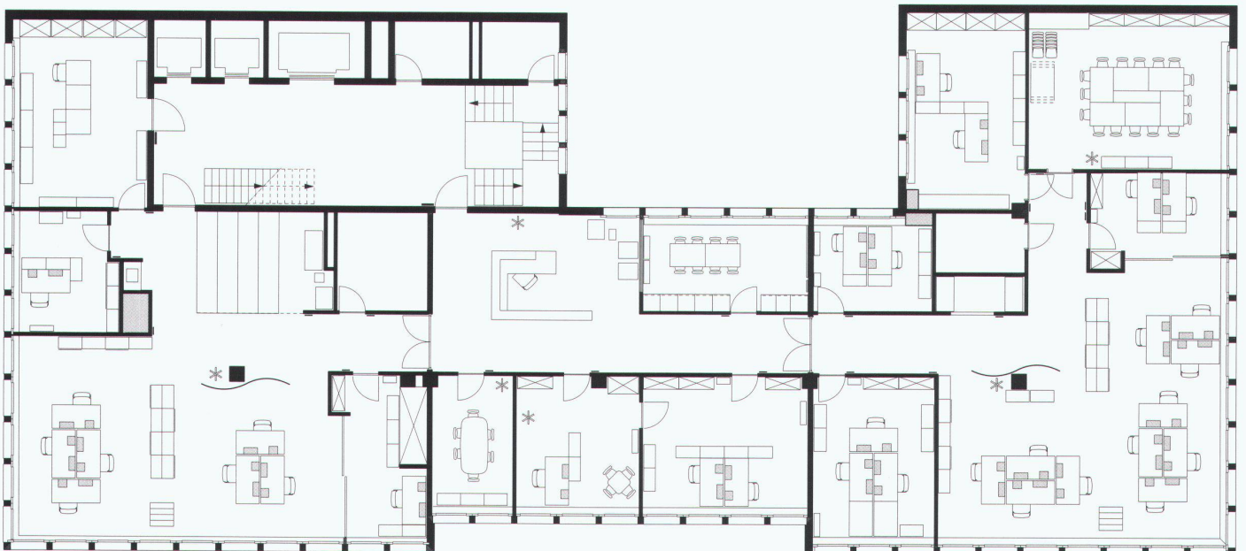
Grundriss
