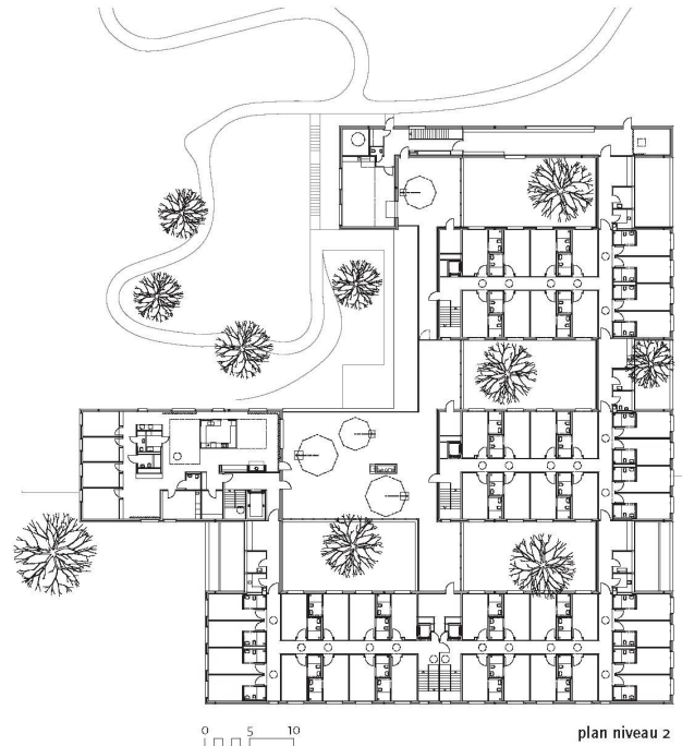
plan niveau 2
