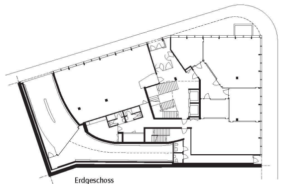
Erdgeschoss
