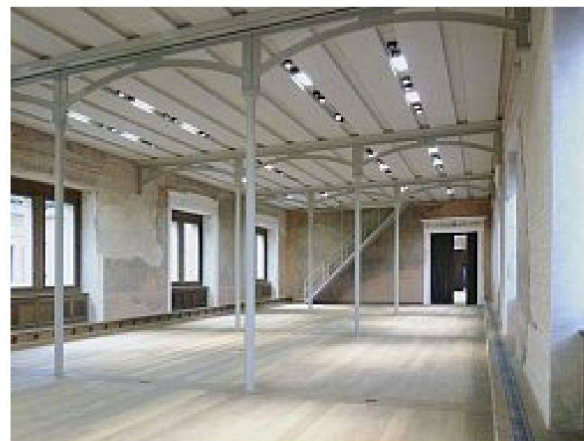
Neue Eisenstützen in den Sälen des 2. Obergeschosses. – Bild: Christian Raabe
