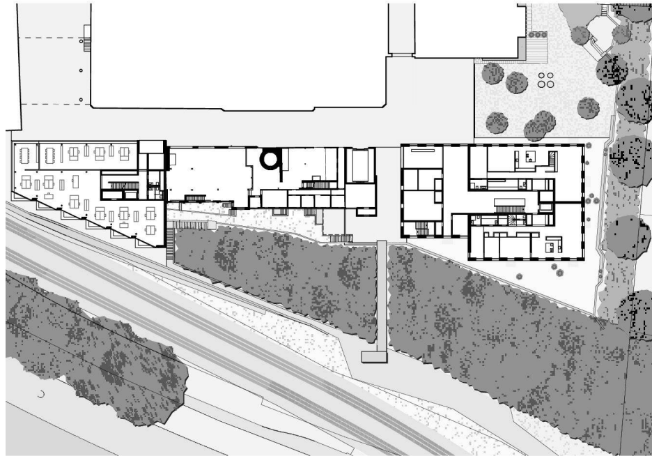
Erdgeschoss Berganlage: links Bürogebäude, rechts Wohngebäude Malturm
