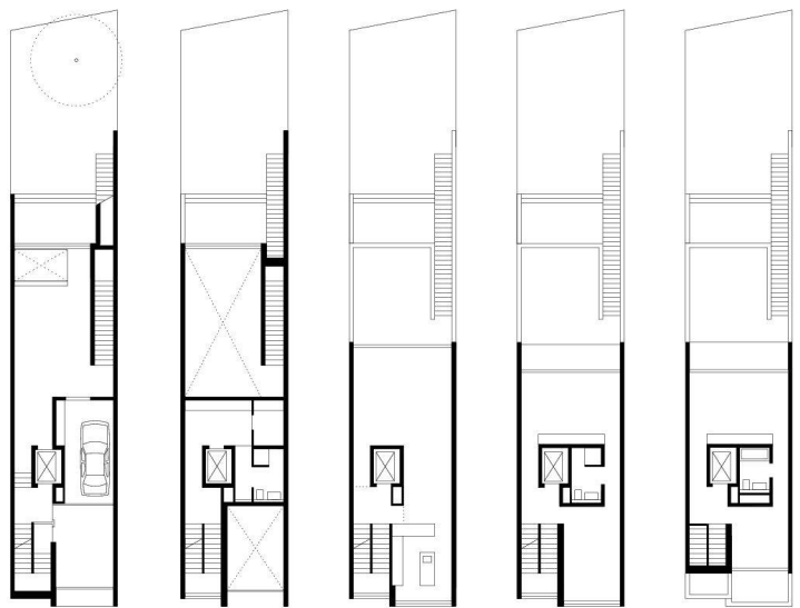
Auf geringer Grundstücksbreite wird die Vertikalität durch die Setzung des Kerns als strukturierendem Element der Geschosse inszeniert.
