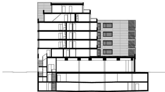
Querschnitt
