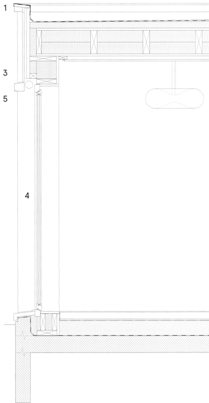
Detailschnitt
