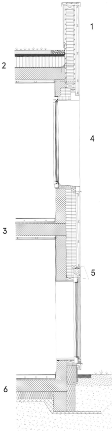
Detailschnitt
