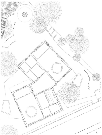
Erdgeschoss
