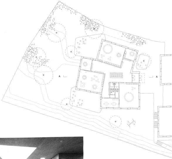
Grundriss
