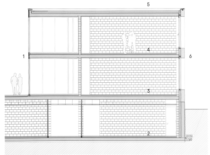
Detaillschnitt
