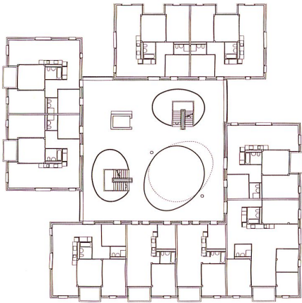
Gebäudegruppe Nord, Normalgrundriss mit grösseren Einheiten
