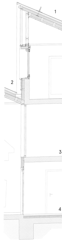
Coupe détail
