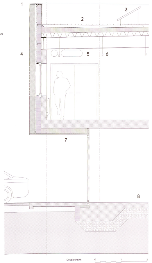
Detailschnitt
