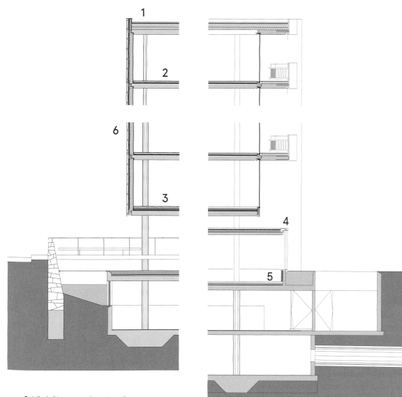
Detailschnitt 0 1 2
