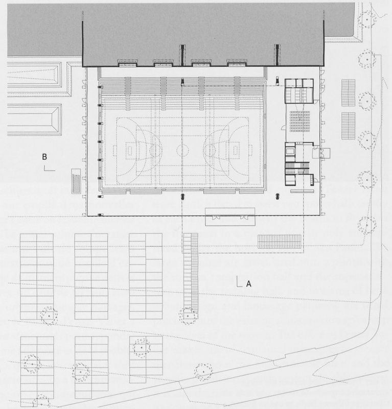
Erdgeschoss
