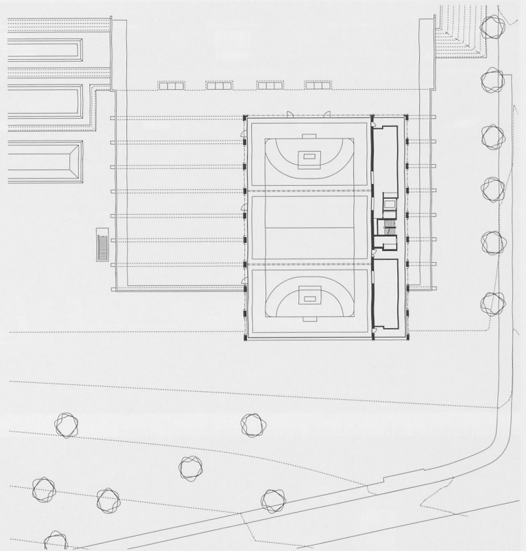
Obergeschoss
