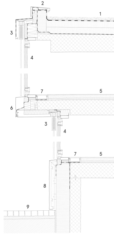
Coupe constructive 0 5
