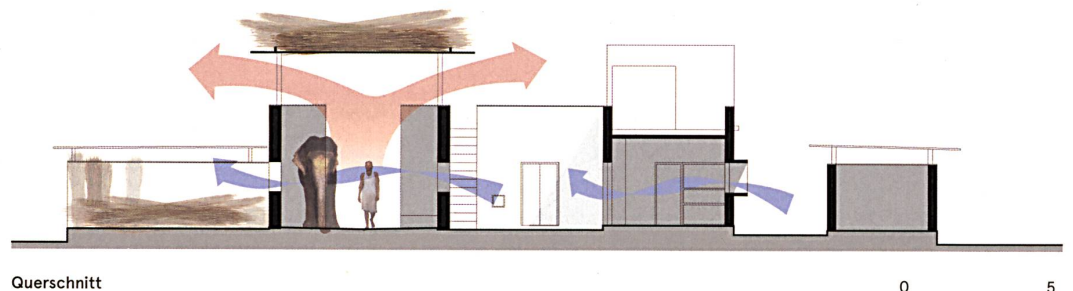
Querschnitt
