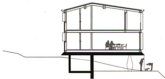
Schnitt
