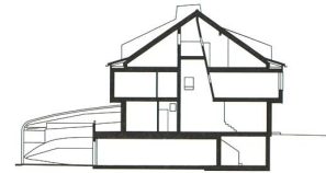
Querschnitt «Flarz 2»
