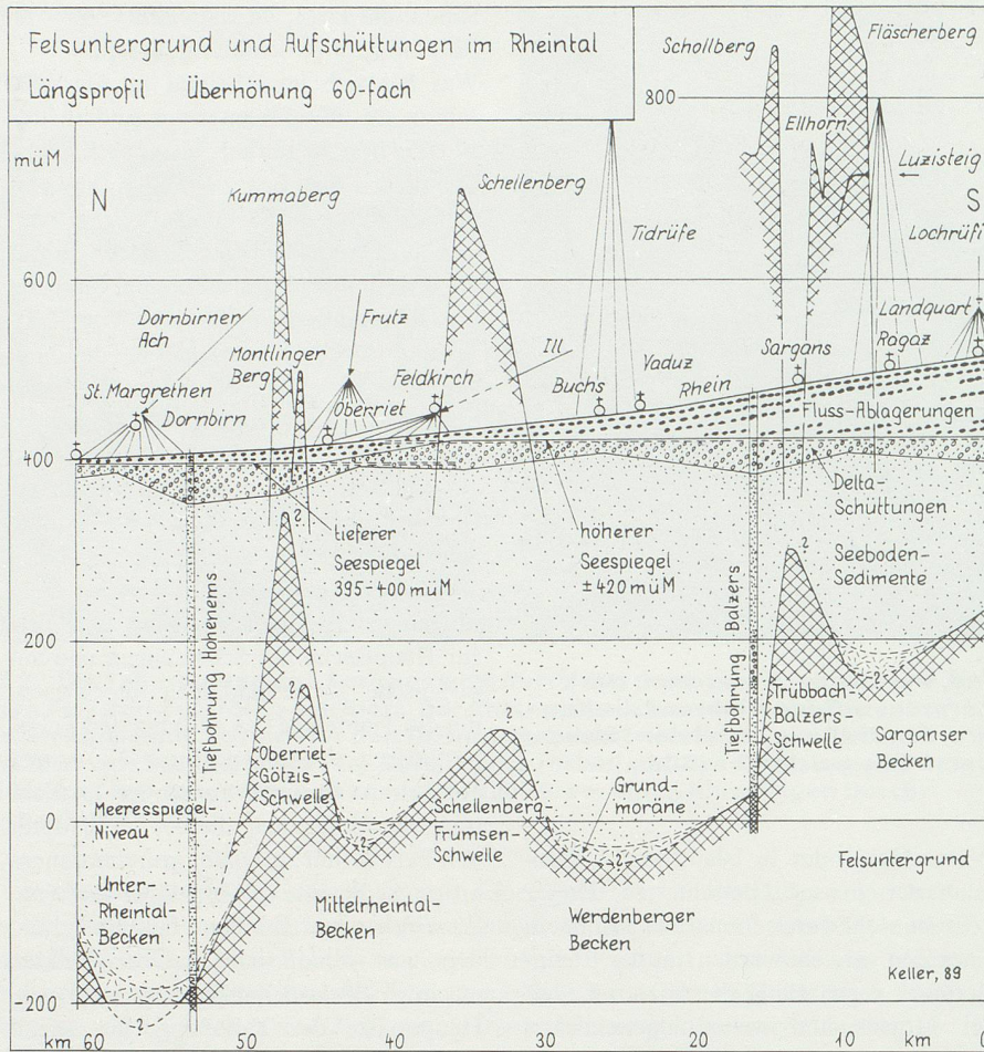
Figur 3: Der Verlauf der Felsoberfläche als eigentlicher Boden des Rheintals weist eine Reihe von Becken und Schwellen auf. Die erstaunliche Tiefe auch noch weit im Alpeninnern zeugt von der grossen Erosionsleistung der Eiszeitgletscher. Gewaltige Mengen an Lockermaterial wurden seit dem Abschmelzen der Gletscher abgesetzt. Die Hauptmassen bilden feine Seesedimente und nicht die erwarteten Flussschotter.
