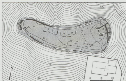
Plan der spätrömischen Hügelsiedlung Carschling bei Castiel im Schanfigg. (Ausgrabung Archäolog. Dienst Graubünden.)
