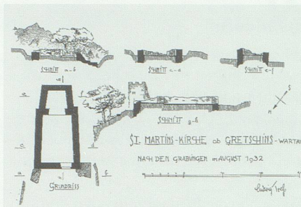
Schnitt und Grundriss der Kapelle auf dem Ochsenberg von Ludwig Tress.
