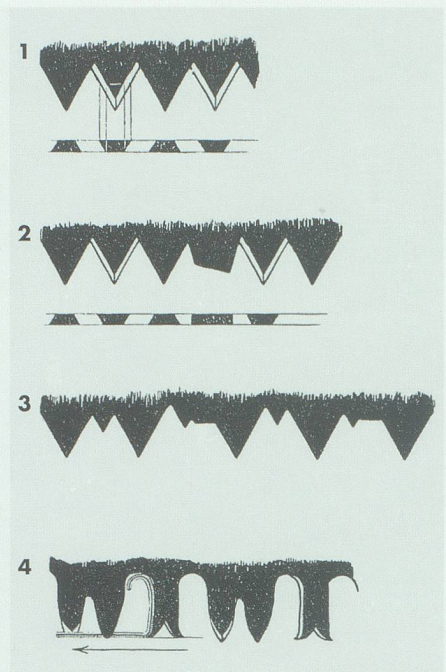
Zahnung des Sägenblattes: 1. Dreieckzahnung; 2. mit Rumer unterbrochene Dreieckzahnung; 3. schlecht nachgefeilte Dreieckzahnung; 4. Hobelzähnsäge mit Schneide- und Hobelzähnen. Bild aus Schmitter 1953.
