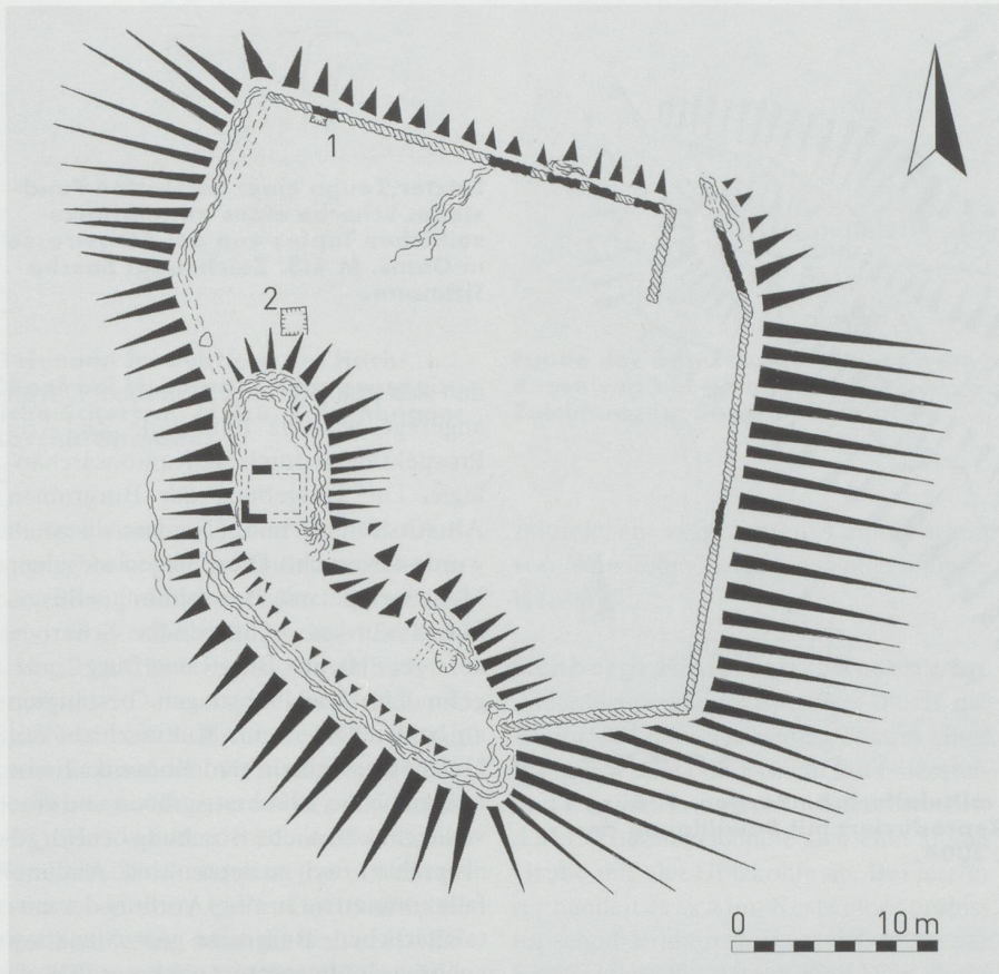
Mittelalterliche und vorgeschichtliche Baureste auf dem Sonnenbühl bei Sevelen(?). Zeichnung: Sascha Tittmann. Reproduziert mit Bewilligung des kant. Vermessungsamtes St.Gallen, 9.11.2004.
