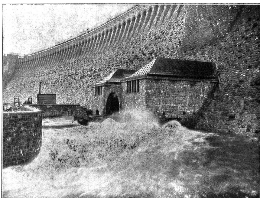
Möhnetalsperre. Abbildung 3. Teilansicht der Sperrmauer. 22 Schieber mit je 1400 mm Lichtweite von Bopp & Reuther, Mannheim.
