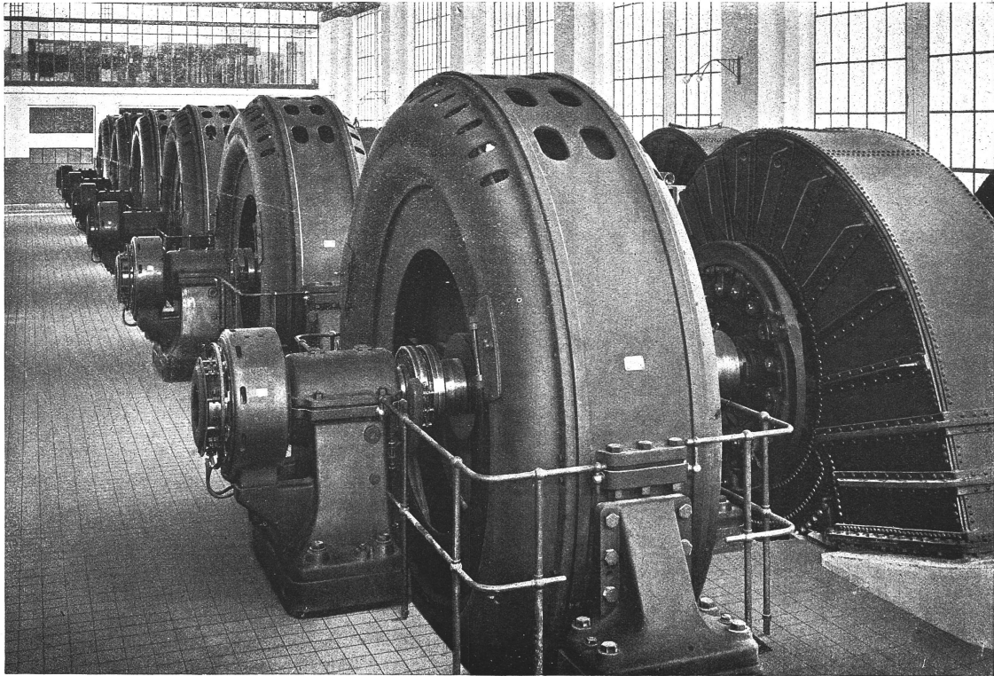
Abb. 42. Elektrizitätswerk Kallnach. Maschinensaal.
