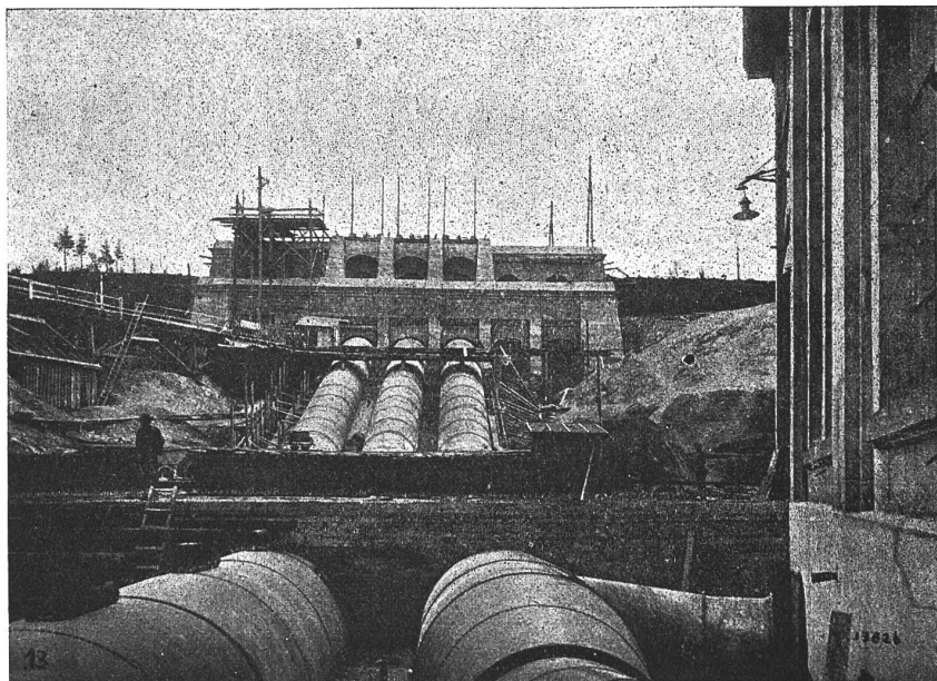
Abb. 37. Elektrizitätswerk Källnach. Wasserschloss und Druckleitungen der Zentrale Källnach im vorgerückten Baustadium.
