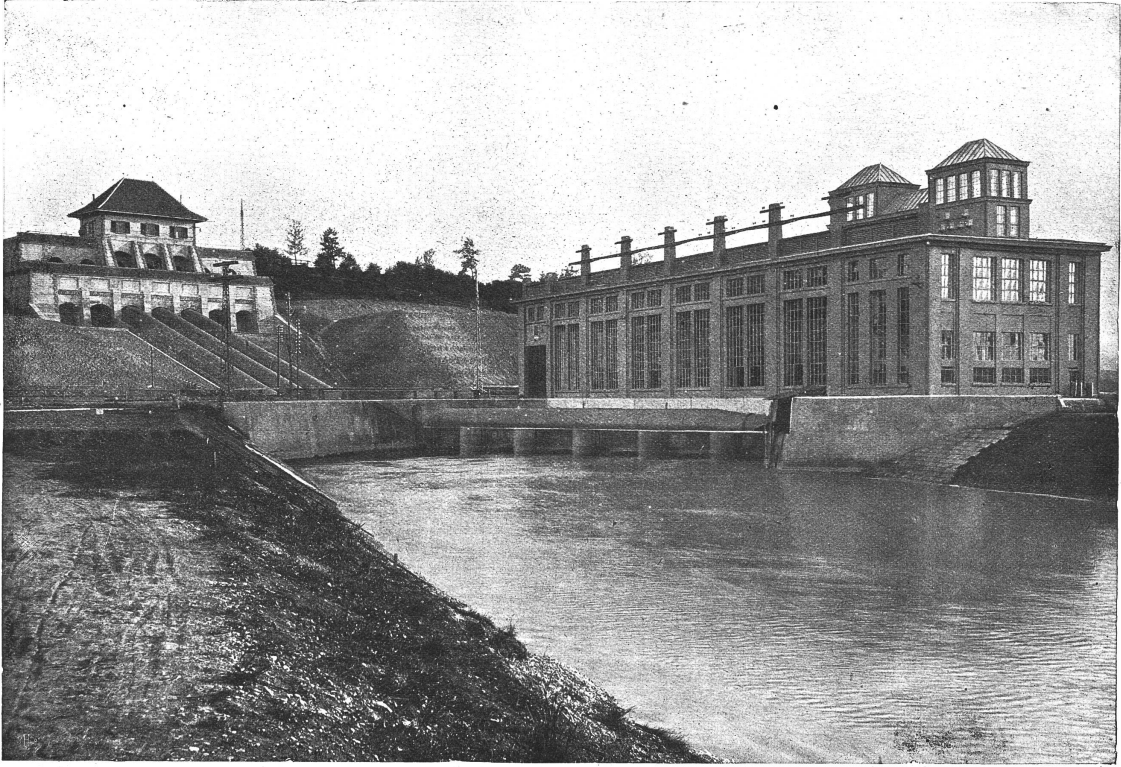
Abb. 40. Elektrizitätswerk Kallnach. Gesamtansicht der Zentrale mit Wasserschloss und Druckleitung von der Unterwasserseite aus gesehen.
