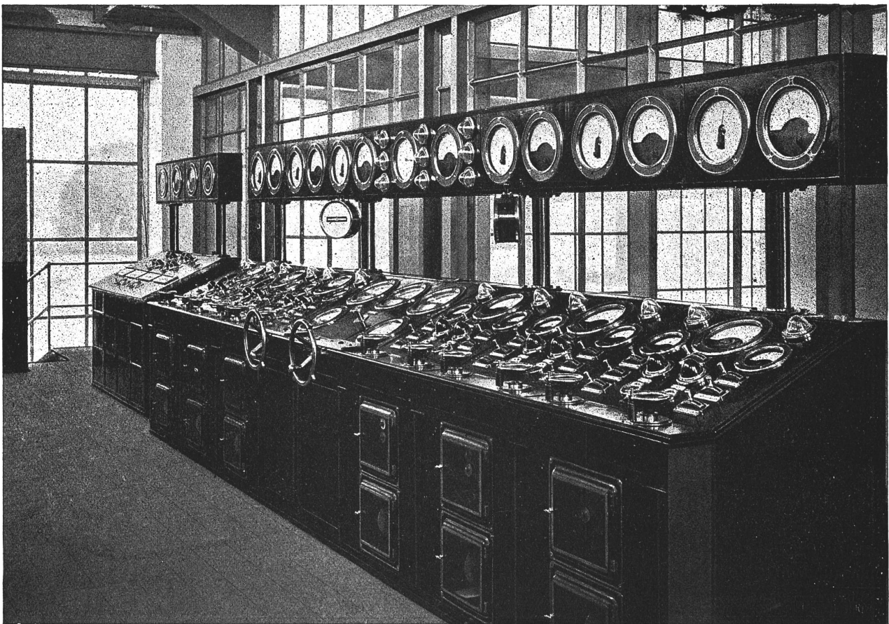
Abb. 44. Elektrizitätswerk Kallnach. Schaltraum (Vorderseite).
