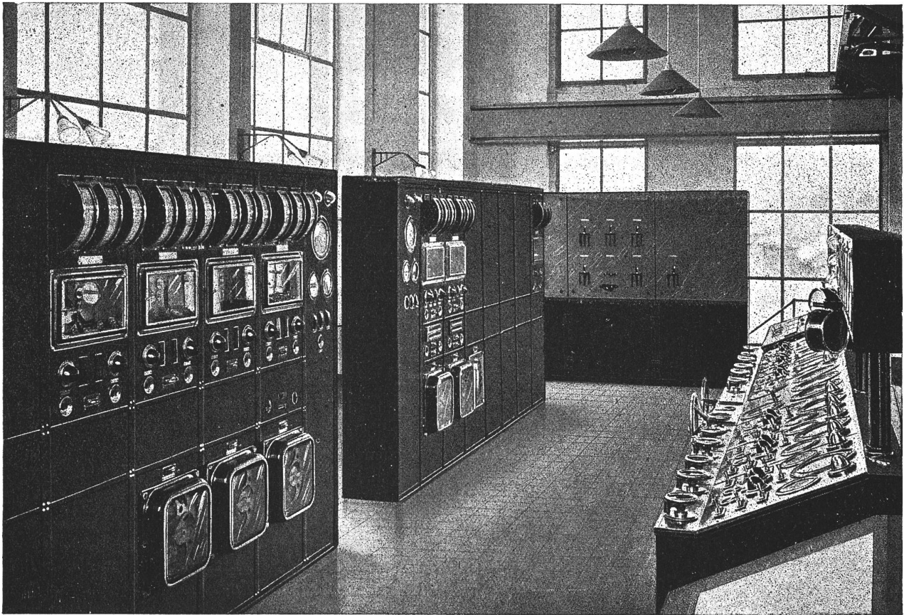
Abb. 43. Elektrizitätswerk Kallnach. Schaltraum (Rückseite).
