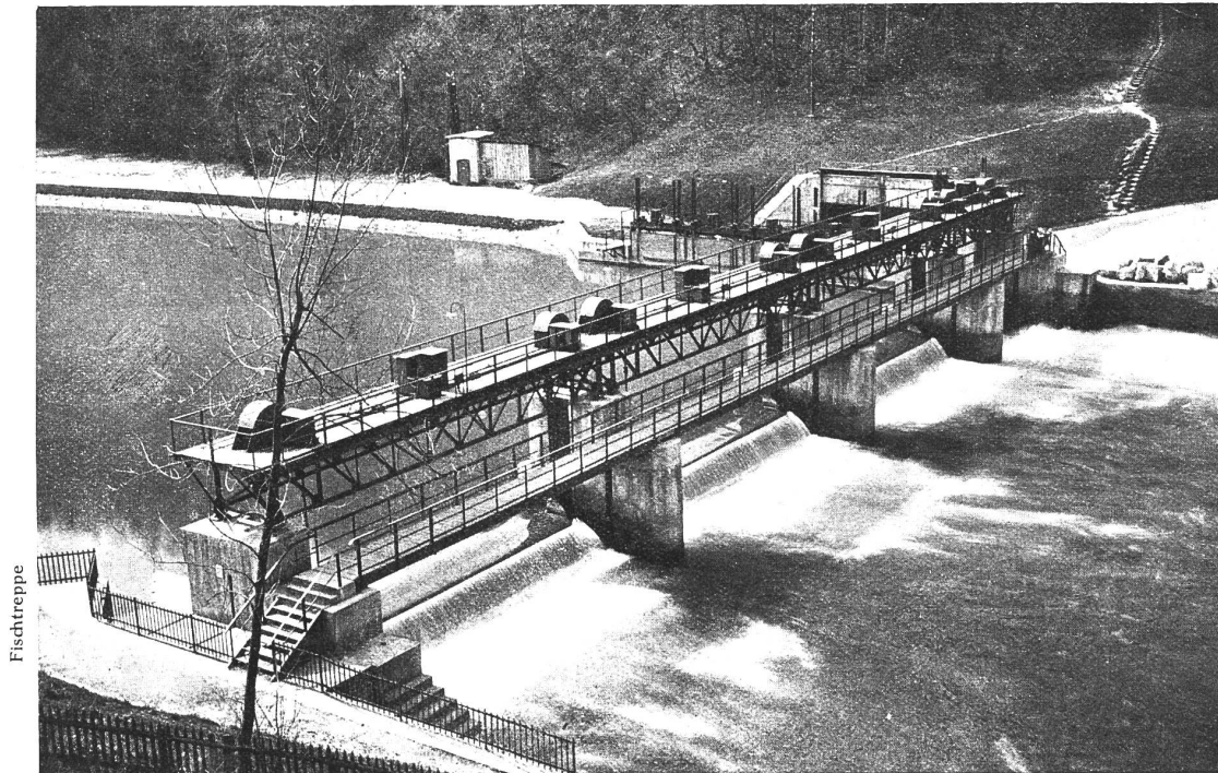
Abb. 26. Elektrizitätswerk Felsenau der Stadt Bern. Stauwehr und Stolleneinlauf, Fischstiege auf dem rechten Ufer
