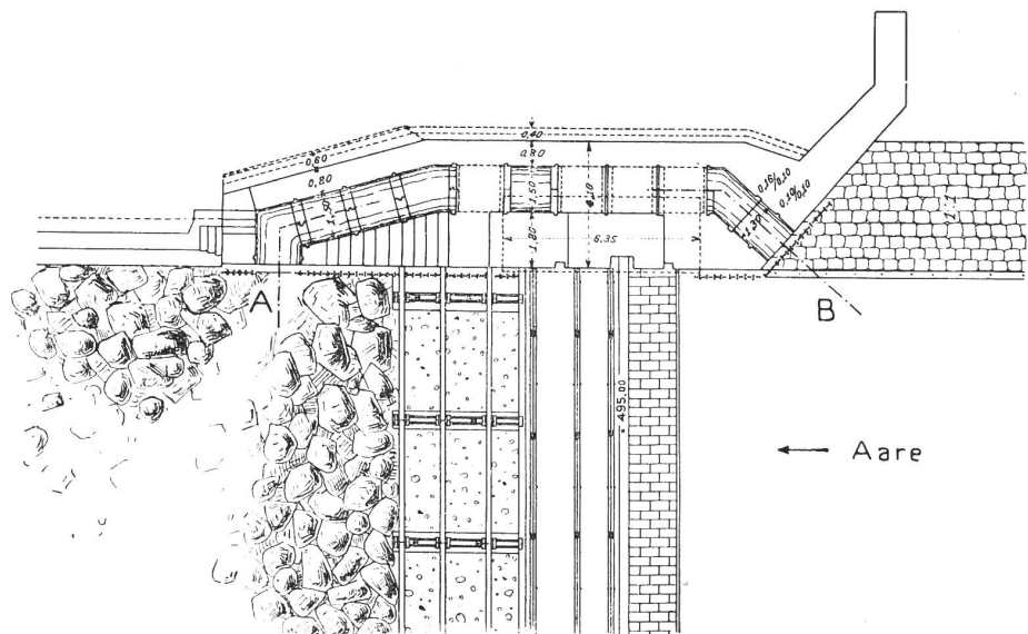
Abb. 27. Stauwehr des Elektrizitätswerks Felsenau der Stadt Bern. Situation der Fischstiege auf dem rechten Ufer. Maßstab 1 : 250.
