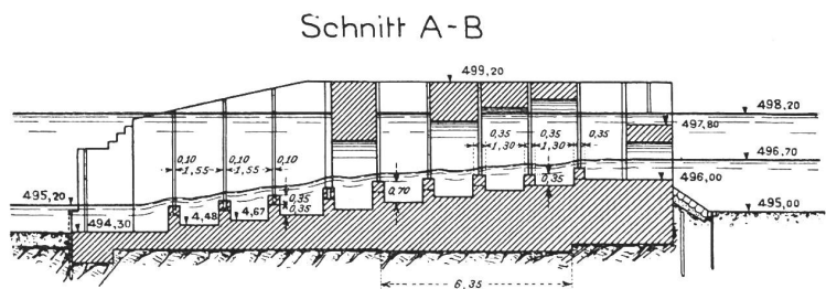
Abb. 28. Stauwehr des Elektrizitätswerks Felsenau der Stadt Bern. Schnitt A — B durch die Fischstiege. Maßstab 1 : 250.
