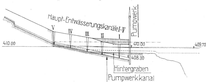
Hintergraben-Pumpwerkkanal. Längen 1 : 100 000, Höhen 1 : 400.
