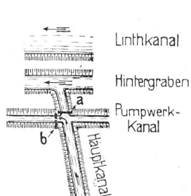
Schützenanordnung.
