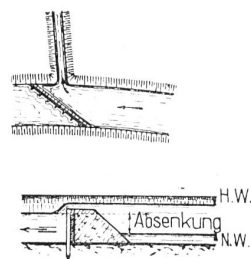
Querschnitte in der Spettlinth und im Böschengießen.
