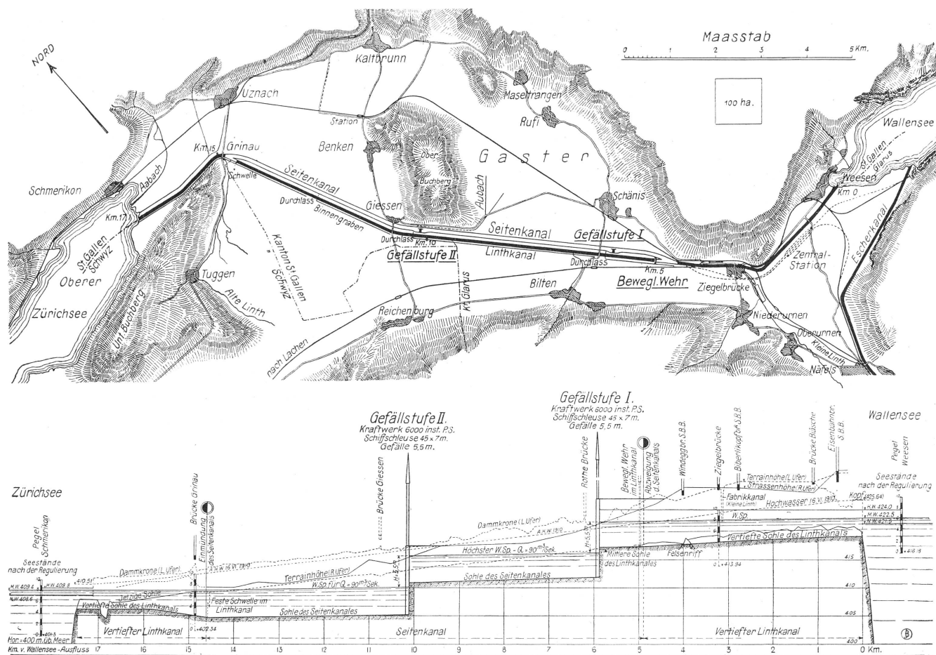
Abbildung 5. Übersichtsplan und Längenprofil des Lint-Seitenkanals. (Projekt Gelpke.)
