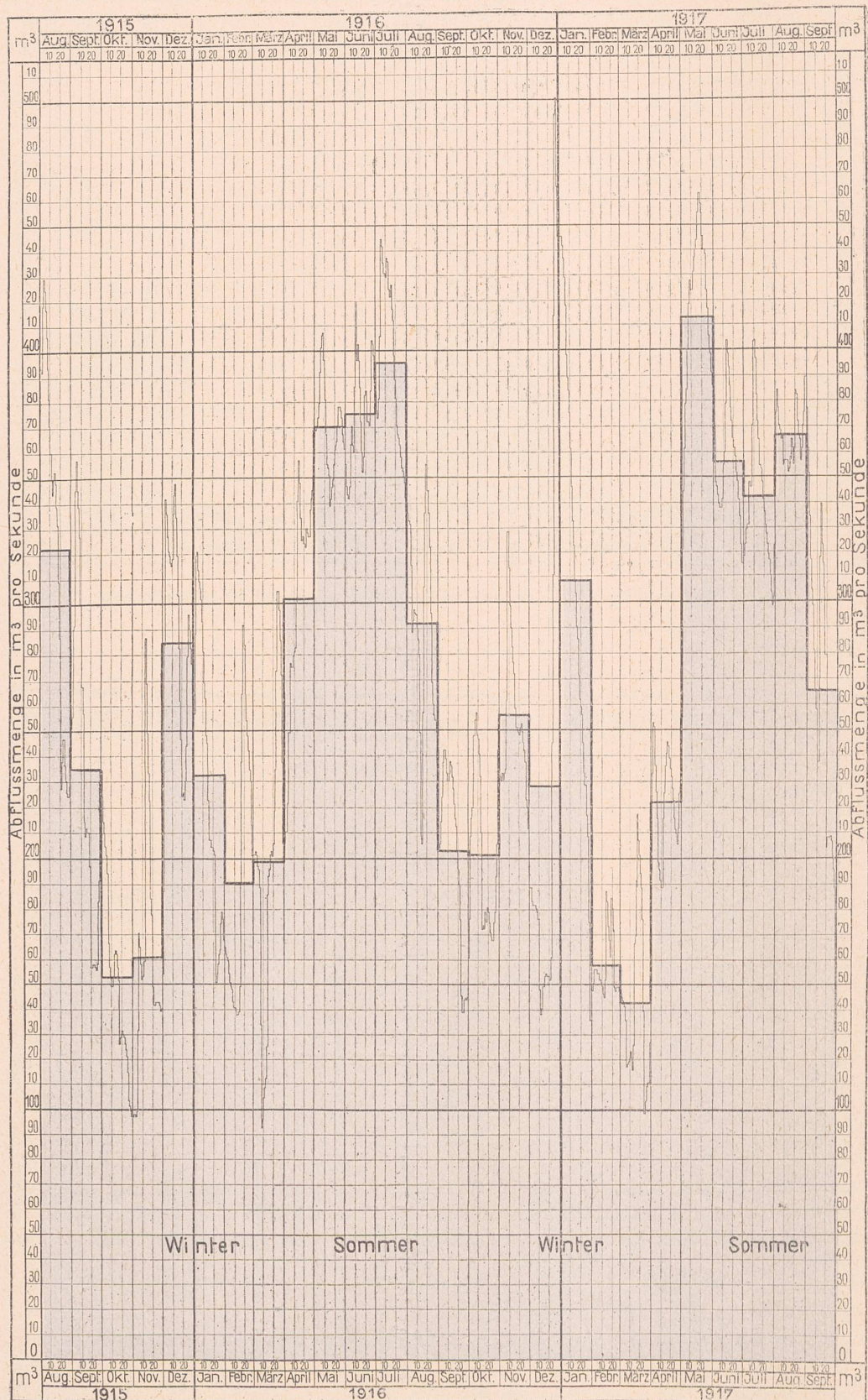
Abb. 7. Tägliche und mittlere monatliche Abflussmengen der Aare bei Brugg von August 1915 bis September 1917.
