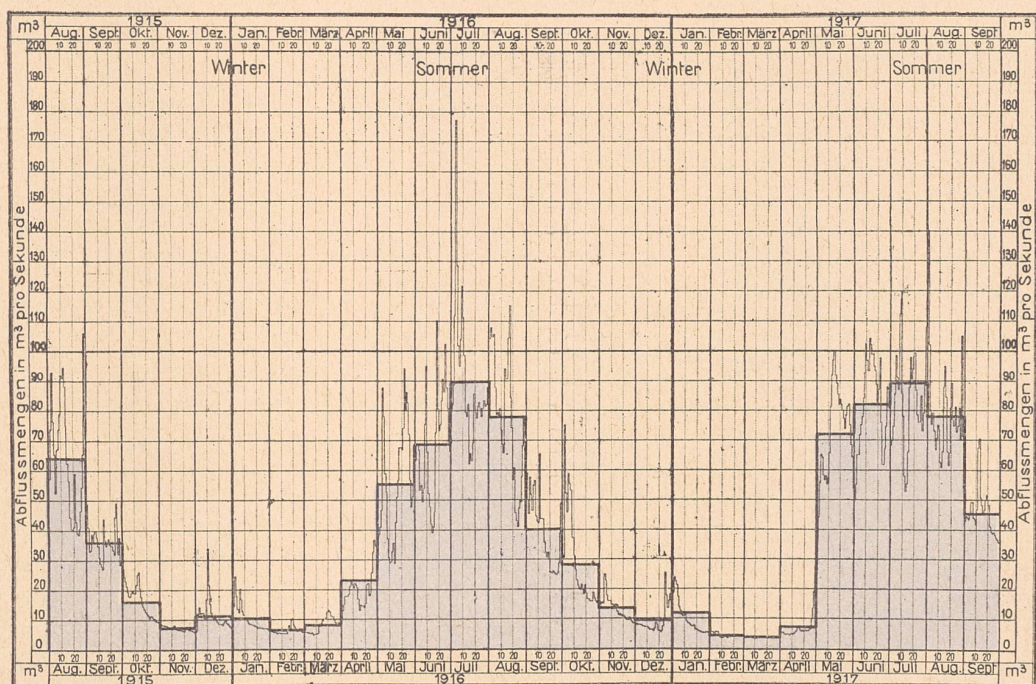
Abb. 5. Tägliche Abflussmengen der Aare bei Brienzwil, August 1915 bis September 1917.
