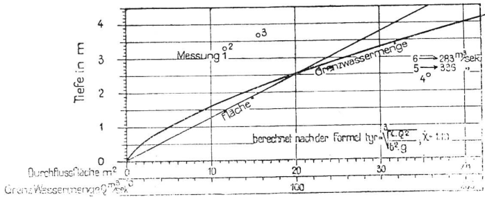
Abb. 7. Grenzwasserabflussmengenkurve im Profil der Schiebepiegel. Distanzzahl 6.40 m.
