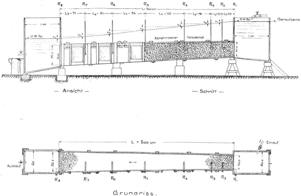
Abb. 1. Versuchskanal zur Ermittlung des Durchfluß-Gesetzes und der Durchlässigkeits-Konstanten für Wasser durch verschiedene Materialien bei verschiedenen Druckhöhen, entsprechend der Formel:
