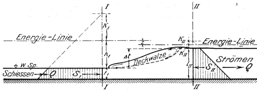
Abb. 12. Darstellung des Wechselsprungs mit Deckwalze. (Die schraffierten Flächen kennzeichnen die Stützkräfte.)
