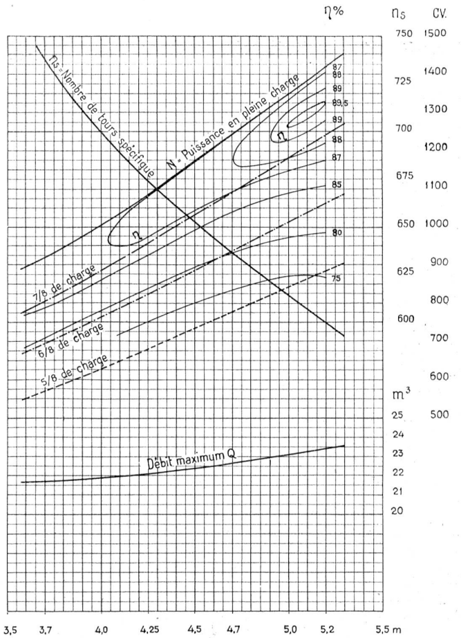
H = Chute nette, en mètres Abb. 4. Leistungsdiagramme der Propellerturbine der alten Centrale Wynau bei den Abnahmeversuchen.
