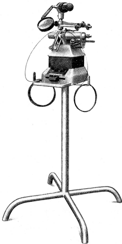
Fig. 13 Elektrischer Feinschweissapparat Appareil à souder électrique de précision (Schlatter & Cie., Zürich).
