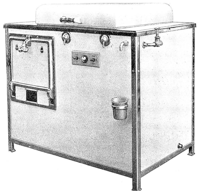
Fig. 9 Pilum-Speicherherd mit 2 Platten, Backofen und Boiler Cuisinière à accumulation «Pilum», à deux plaques, four et réservoir d'eau chaude (A.G. der Eisen- und Stahlwerke vorm. Georg Fischer, Schaffhausen.)
