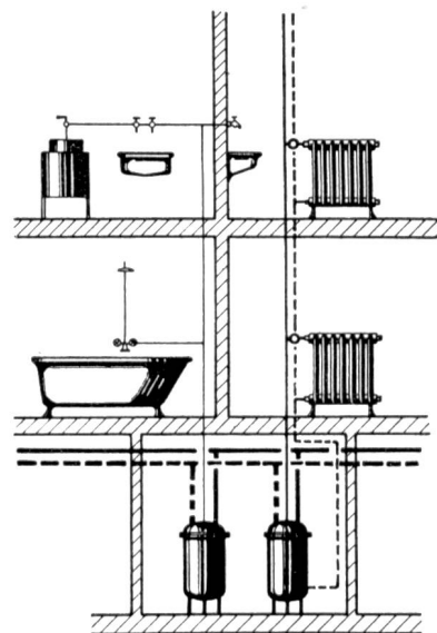
Fig. 24 Schema einer Unterstation. Schéma d'une sous-station. — Vorlauf Aller { Heisswasser — Eau surchauffée - - - Rücklauf Retour { — Vorlauf Aller { Warmwasserh. — Chauffage à eau chaude - - - Rücklauf Retour { - - - Gebrauchswarmwasser — Eau chaude ménagère
