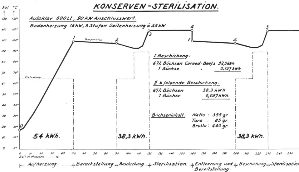
Fig. 8 Arbeits- und Temperatur-Diagramm der Konserven-Sterilisation. Diagramme de la stérilisation des conserves.
