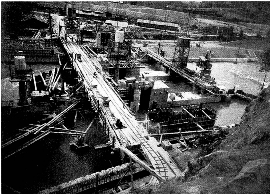
Fig. 26 Evionnaz. Le Barrage. — Vue aérienne de la rive droite. Le 14 mai 1948. Il reste deux caissons en forçage. La superstructure des piles est en construction. Au 1 er plan, la prise d'eau et le pont de service principal. La passe 3 est en eau, mais n'est pas encore libérée.
