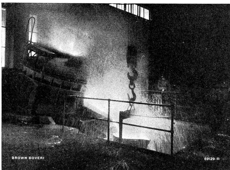
5-t-Elektro-Schmelzofen
