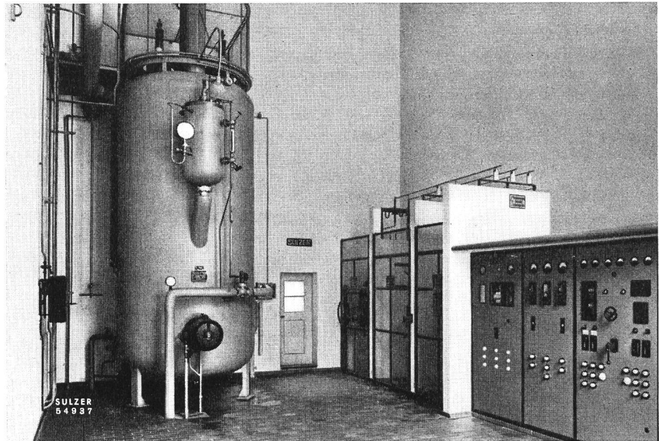
Sulzer - Hochspannung - Elektrokesselanlage von 4000 kW, 12 000 Volt, 13 atü Betriebsdruck, in einem chemischen Werk.
