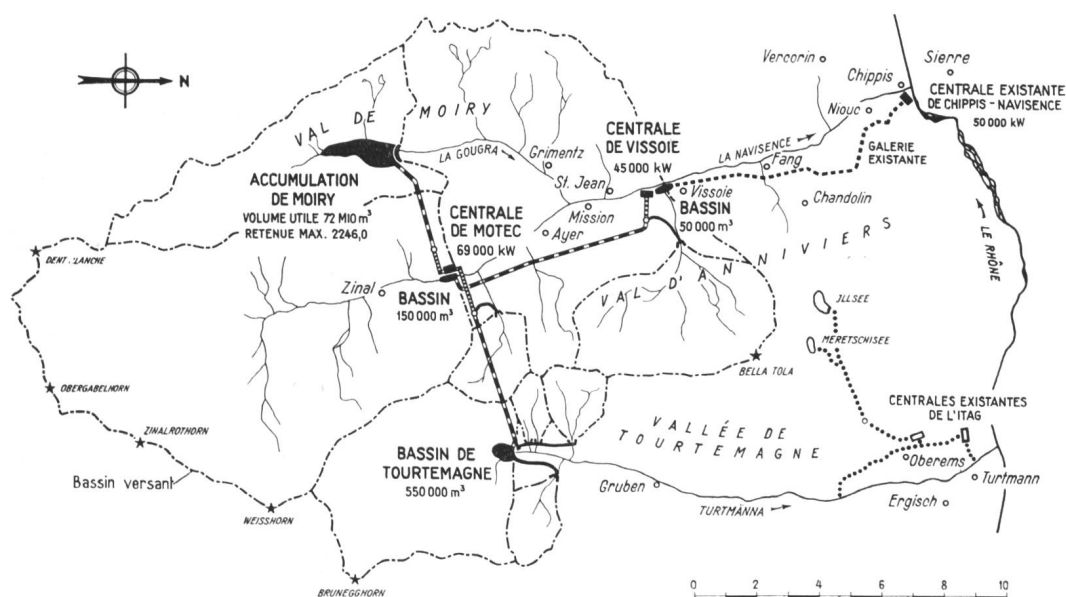
Abb. 1 Kraftwerke Gougtra, Gesamtanlageplan 1 : 250 000
